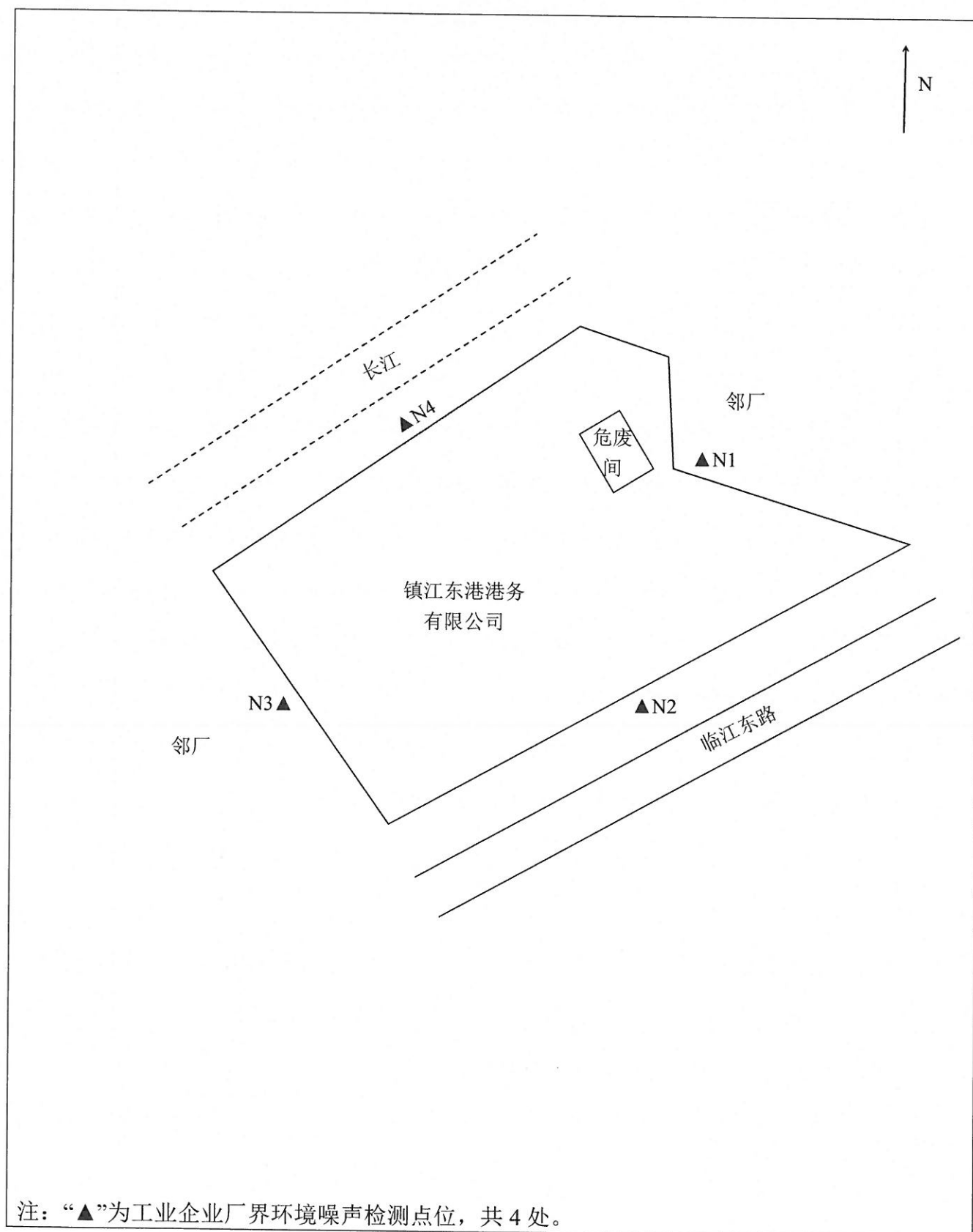
检测点位示意图
